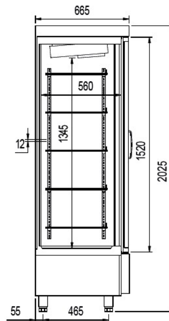
ARPA-ARA-ARAC-125
